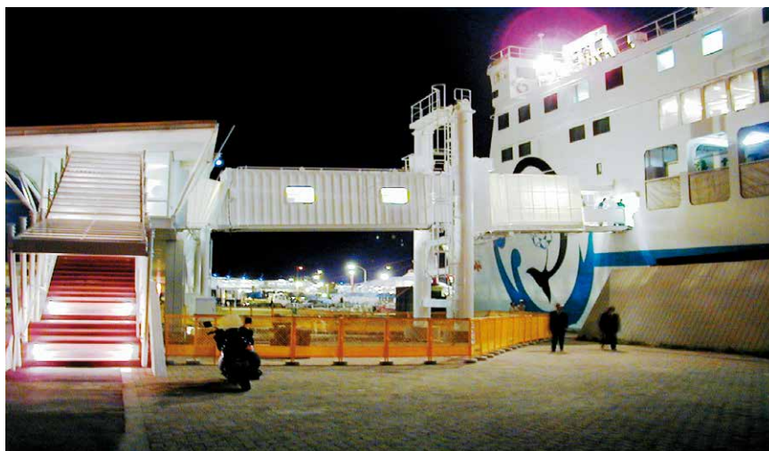
松山港人道橋(ギャングウェイ装置)
