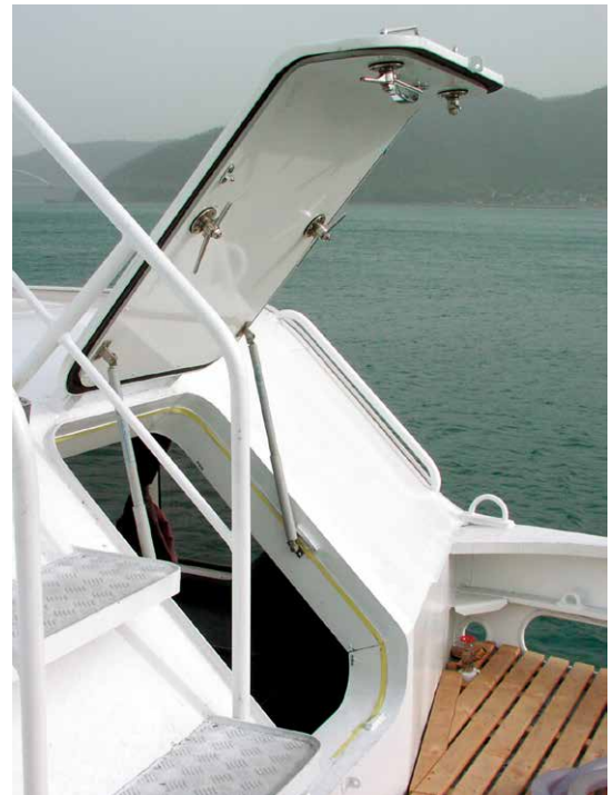
(右)変型部に合わせて製作された水窓ガルウイングドア
